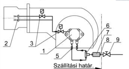
Hárompont szabályzás. O3/2
