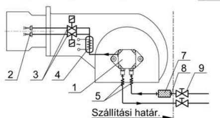
Hárompont szabályzás előmelegítővel. O3R
