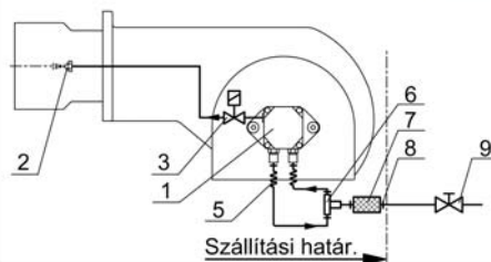
Kétpont szabályzás előmelegítővel. O2R
