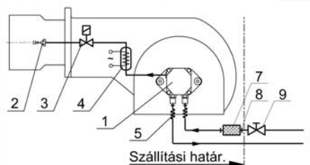
Hárompont szabályzás. O3/1
